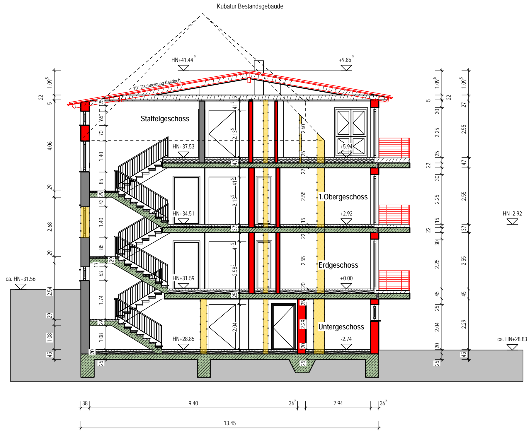
Schnitt A-A
